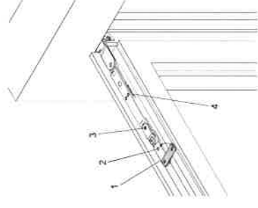
Bild 2: Schere
