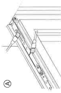
Bild 1: Schere (Flügel)
